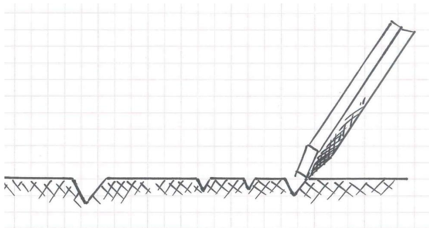
Heraus Arbeiten des Reliefs bzw. der Schrift in Keilform mit 6 mm Schriftmeissel
