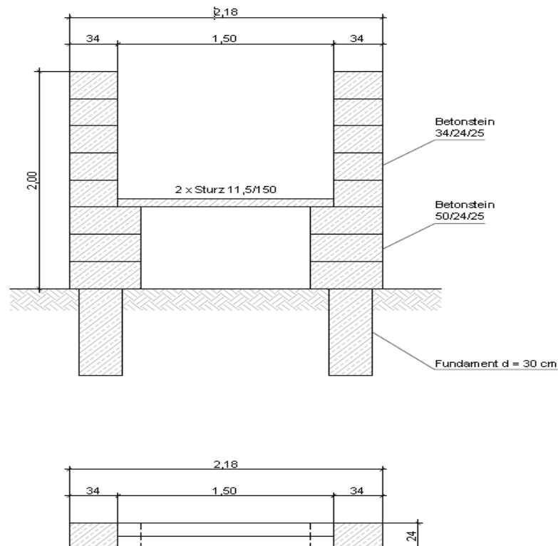
Insektenhotel M 1 : 25
